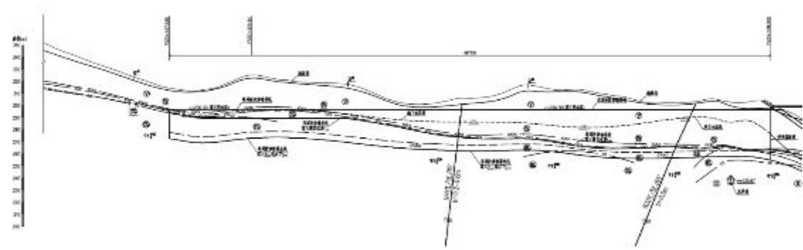
图 6.2-6 下水库大坝左岸库周防渗纵剖面布置图
