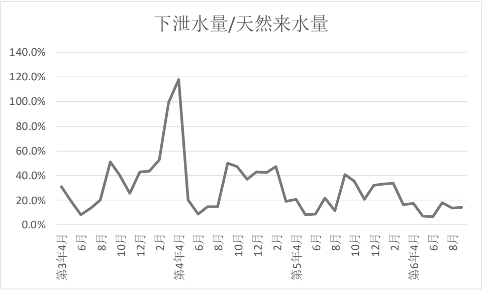
图 6.1-8 蓄水期下水库下泄水量与天然来水量占比
