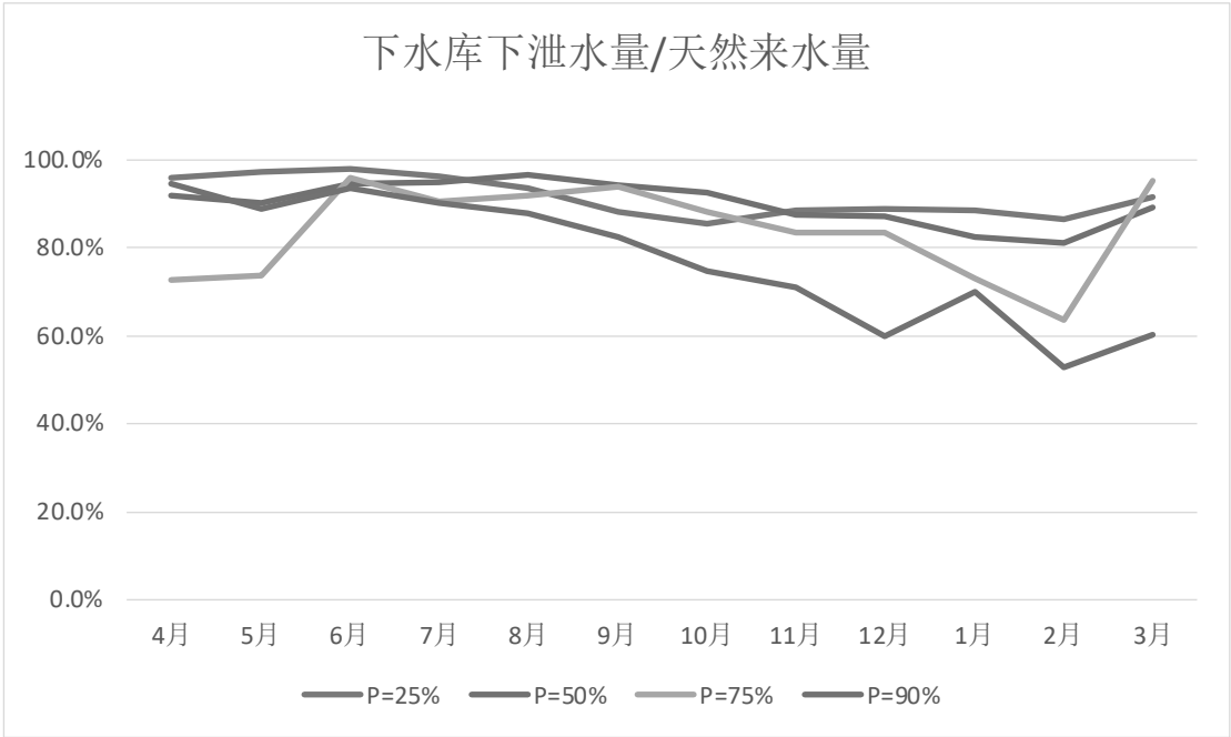
图 6.1-5 施工期下水库各典型年下泄水量占天然来水量比例
