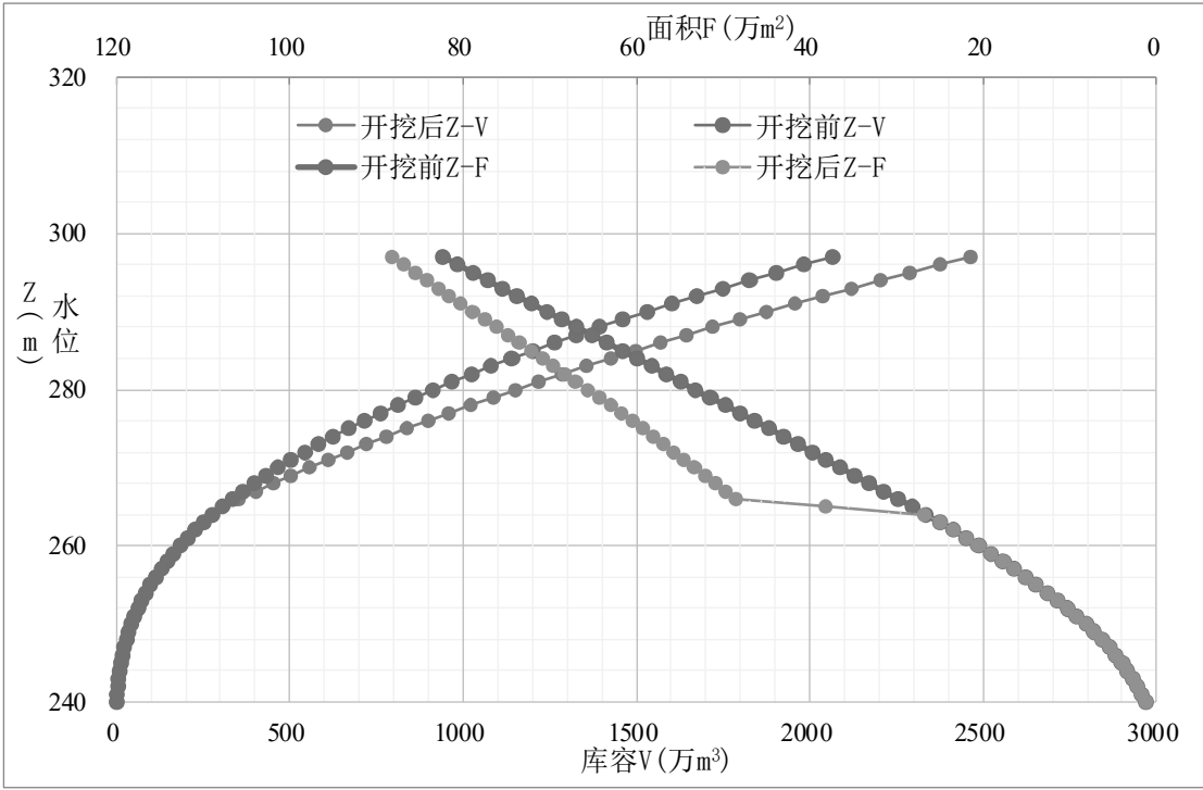
图 6.1-14 下水库水位-水面面积-库容曲线
