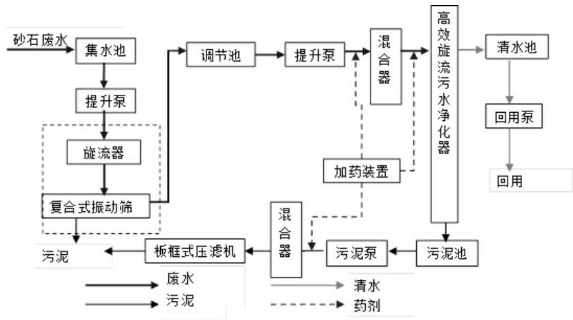
图 8.2-1 高效(旋流)污水净化法处理流程图
