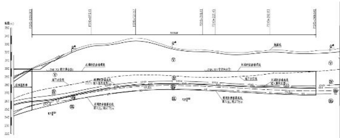
图 6.2-7 下水库大坝右岸库周防渗纵剖面布置图
