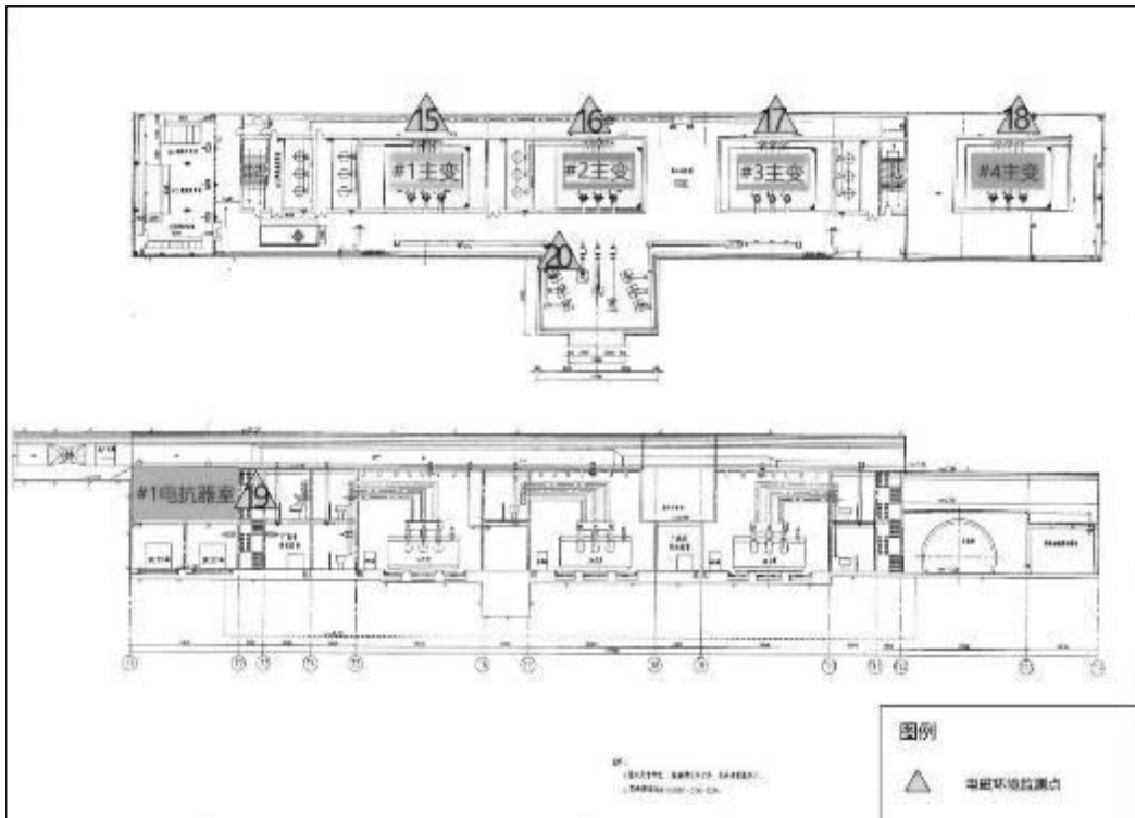
图6.10-3 类比清远市抽水蓄能主变洞电磁环境监测布点图
