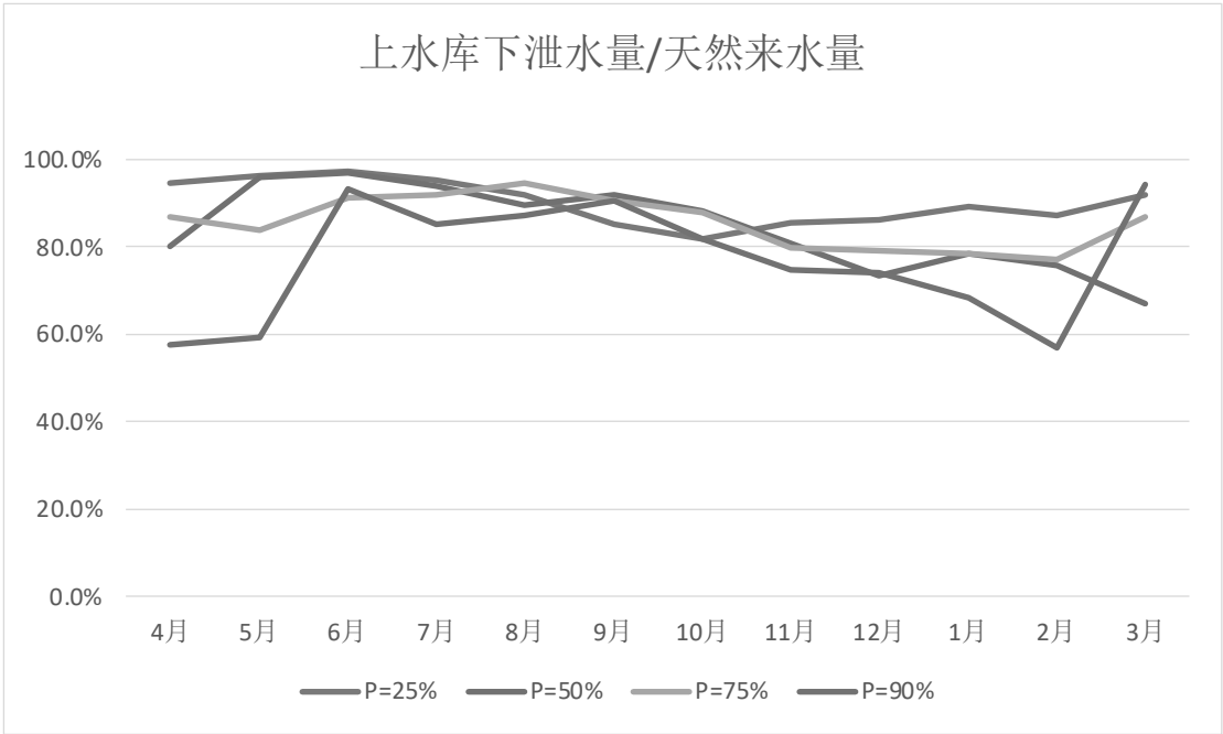
图 6.1-3 施工期上水库各典型年下泄水量占天然来水量比例
