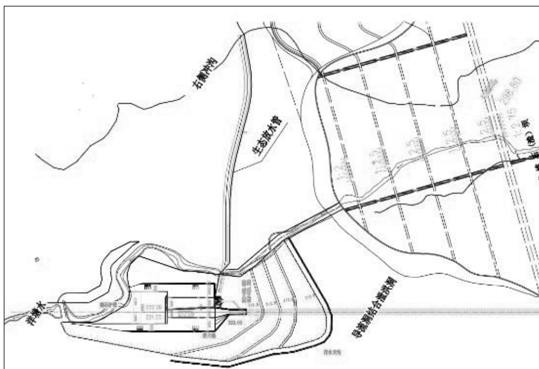
图 8.2-7 下库生态流量管布置示意图
