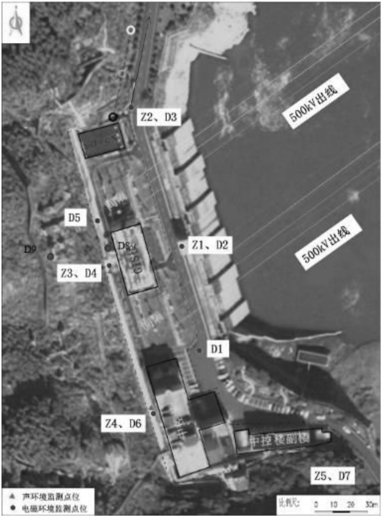
图6.10-4 类比工程开关站电磁环境监测布点图
