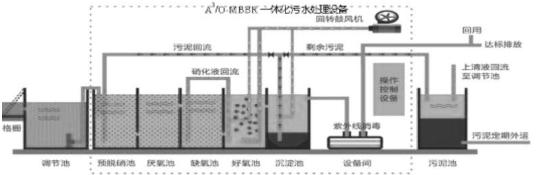
图 8.2-5 施工区生活污水处理工艺流程图
