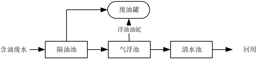
图 8.2-3 机修、汽修废水处理系统工艺流程示意图
