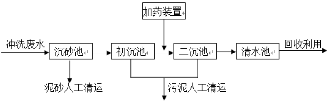
图 8.2-2 混凝沉淀法处理流程图
