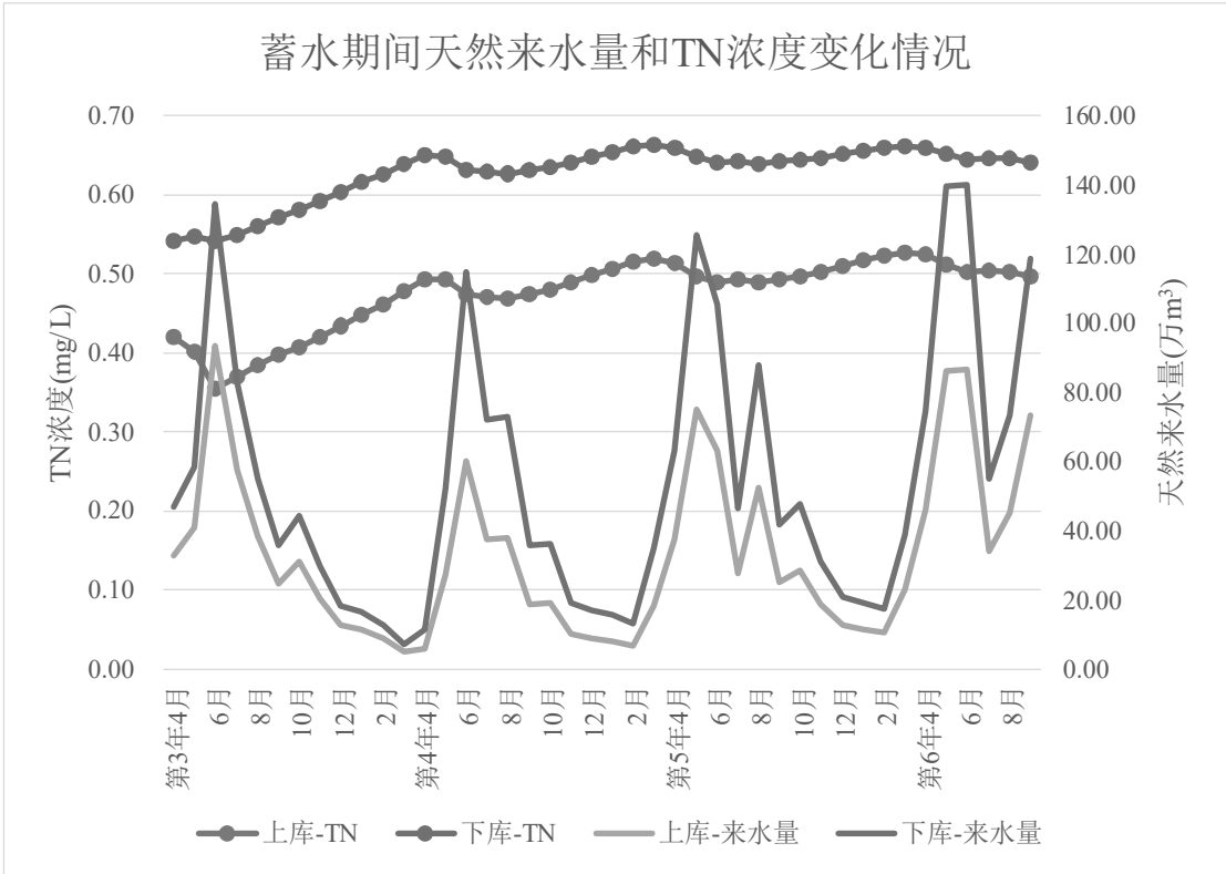
图 6.2-2 蓄水期间上、下水库天然来水量和库区 TN 浓度变化情况
