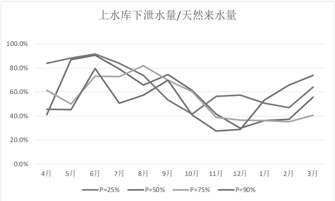
图 6.1-9 运行期上水库下泄水量与天然来水量占比
