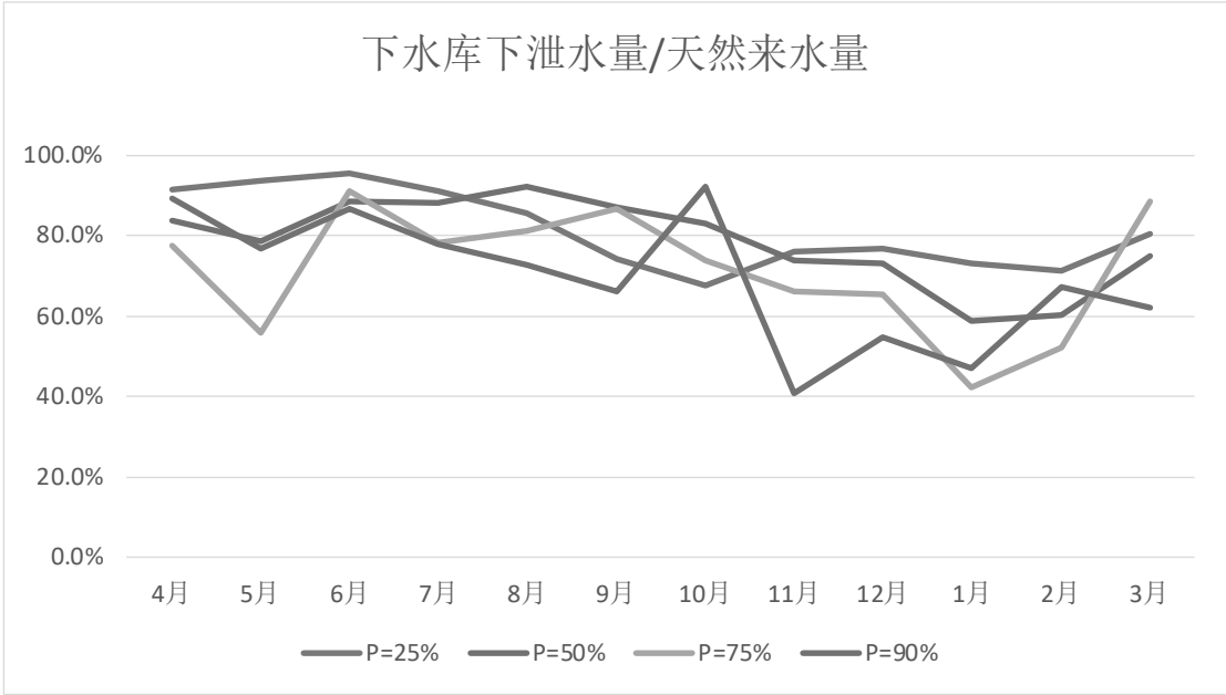
图 6.1-11 运行期上水库下泄水量与天然来水量占比
