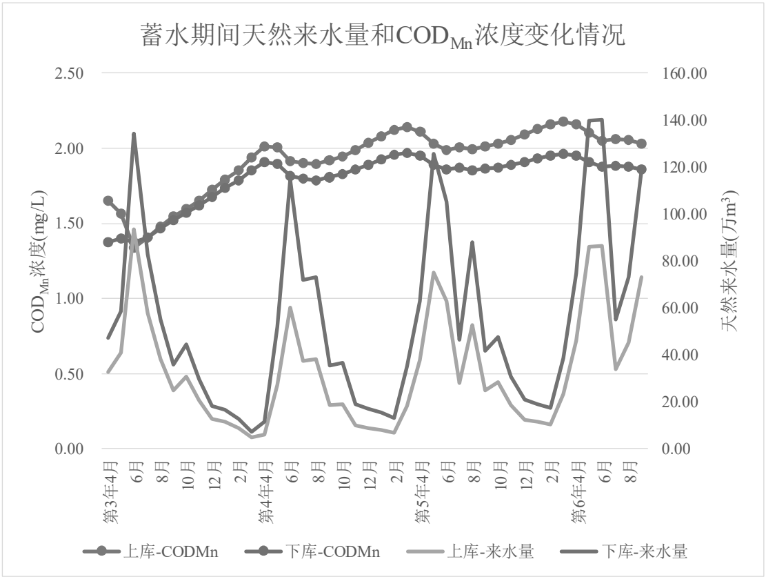
图 6.2-1 蓄水期间上、下水库天然来水量和库区 COD Mn 浓度变化情况
