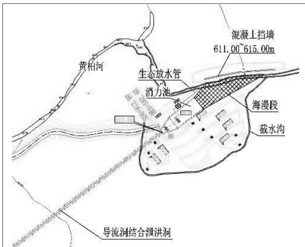
图 8.2-6 上库生态流量管布置示意图
