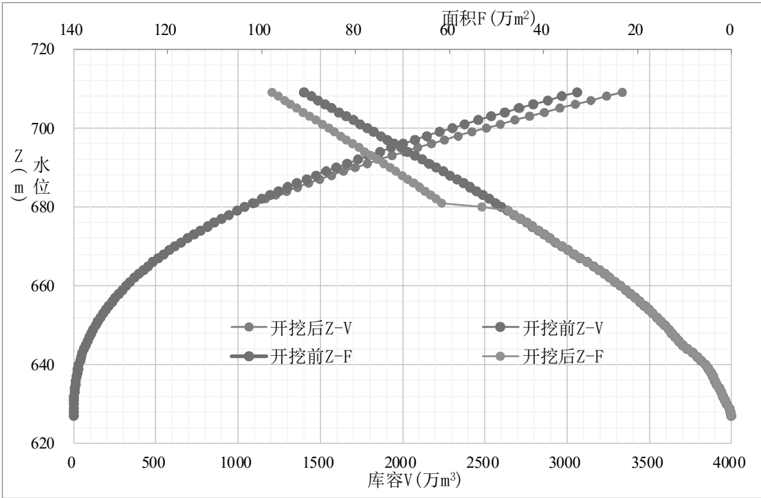
图 6.1-13 上水库水位-水面面积-库容曲线
