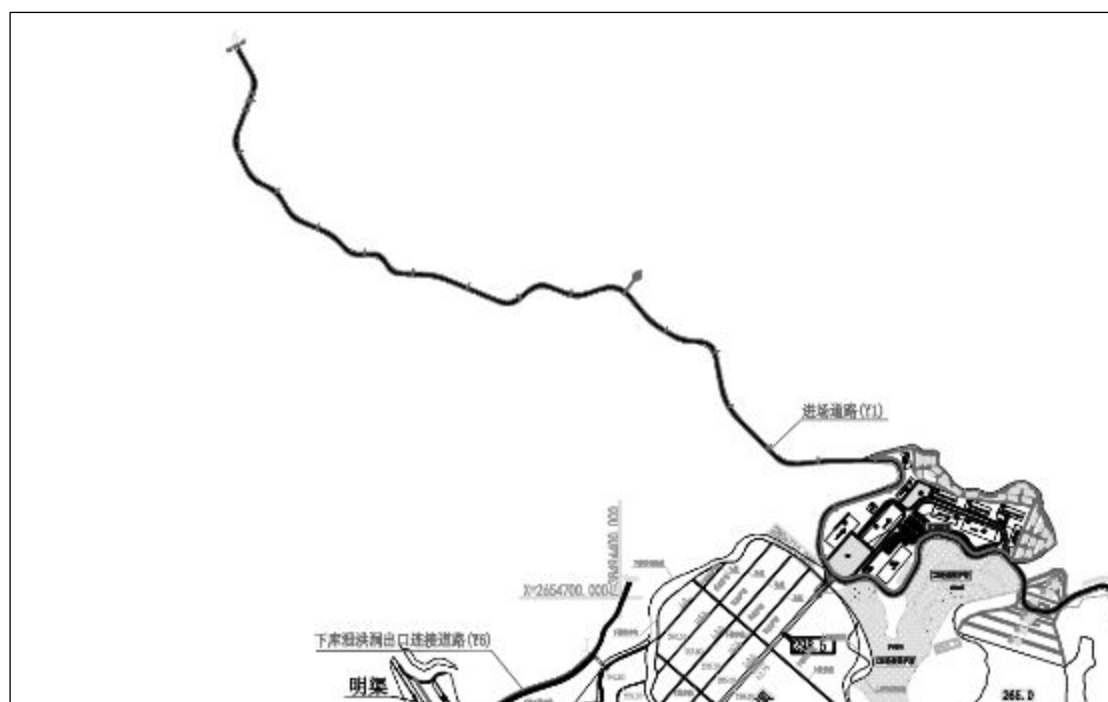
图 2.5-1 进场道路路线方案示意图
