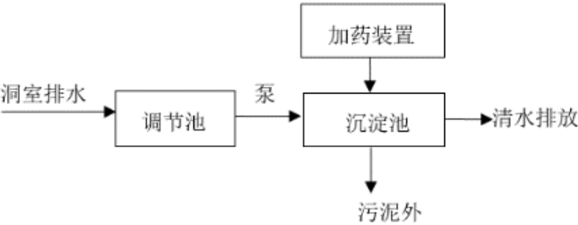
图 8.2-4 洞室排水处理工艺流程图
